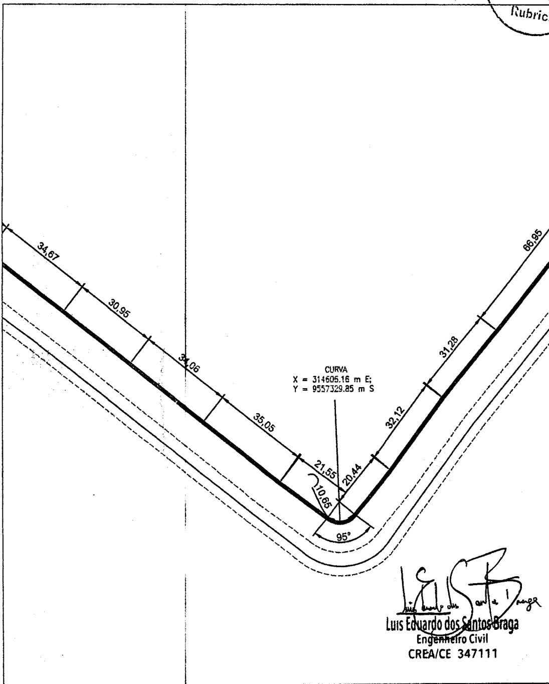
04 PLANTA GERAL (DETALHE 2) ESCALA 1/1150
