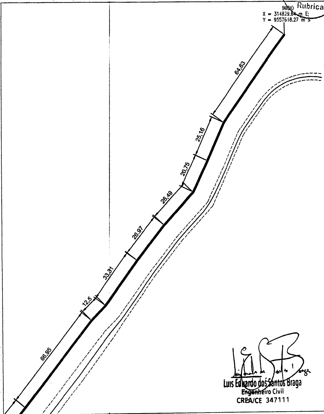
03 PLANTA GERAL (DETALHE 1) ESCALA 1/1150
