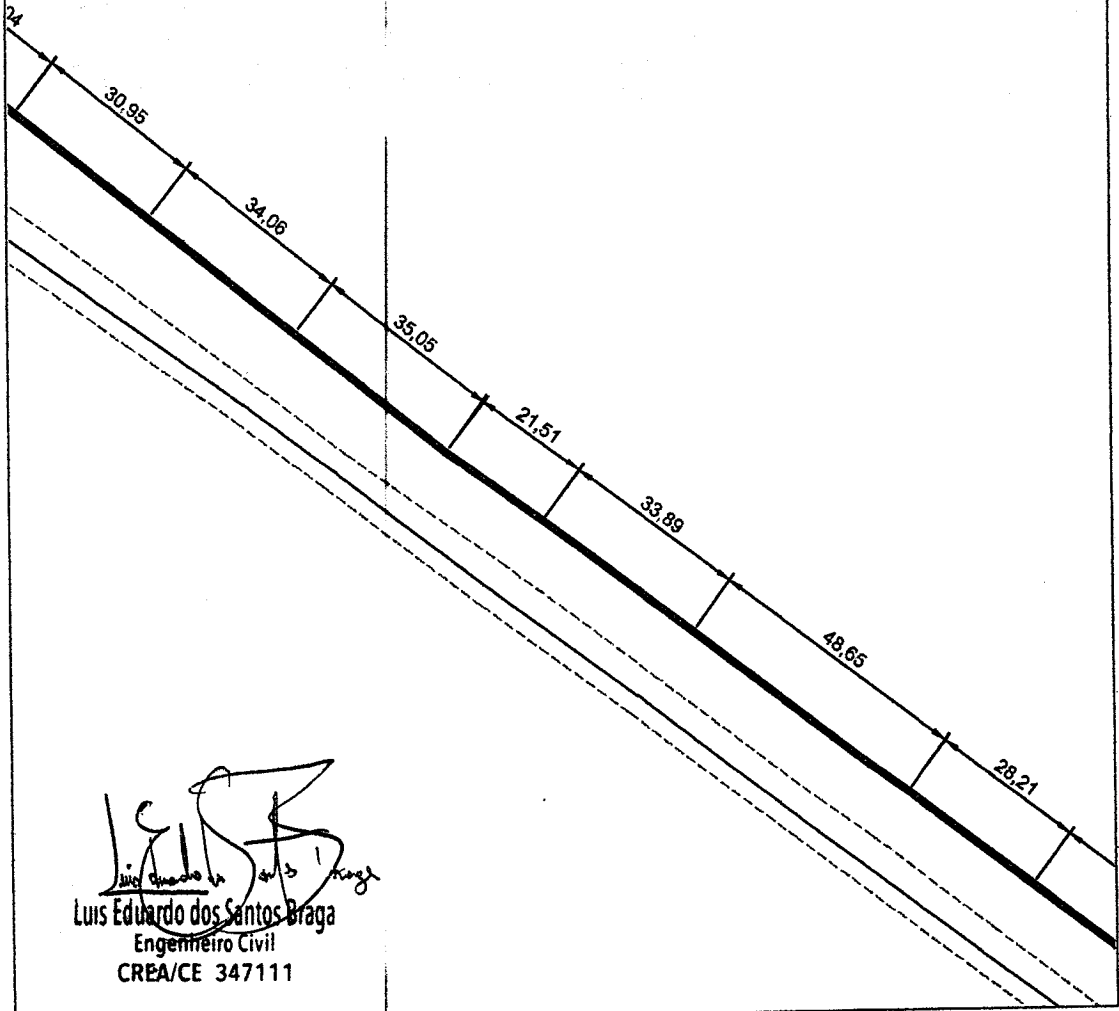
05 PLANTA GERAL (DETALHE 3) ESCALA 1/1150
